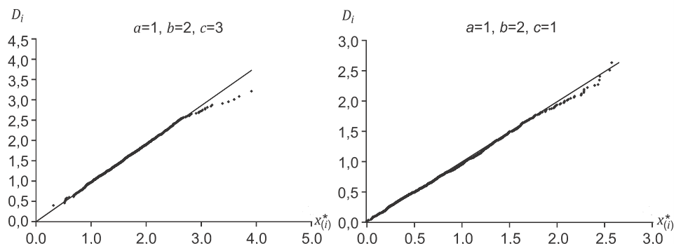
WYKR. 6. SIATKA PRAWDOPODOBIENSTWA URG UZYSKANA METODĄ III
