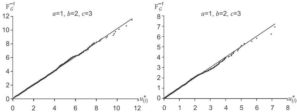
WYKR. 5. SIATKA PRAWDOPODOBIENSTWA URG UZYSKANA METODĄ II
