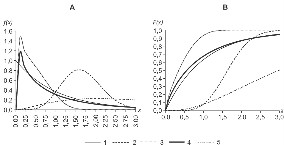
WYKR. 2. FUNKCJA GĘSTOŚCI (A) I DYSTRYBUANTA (B) WYBRANYCH RÓŻKŁADÓW Z RODZINY URG
